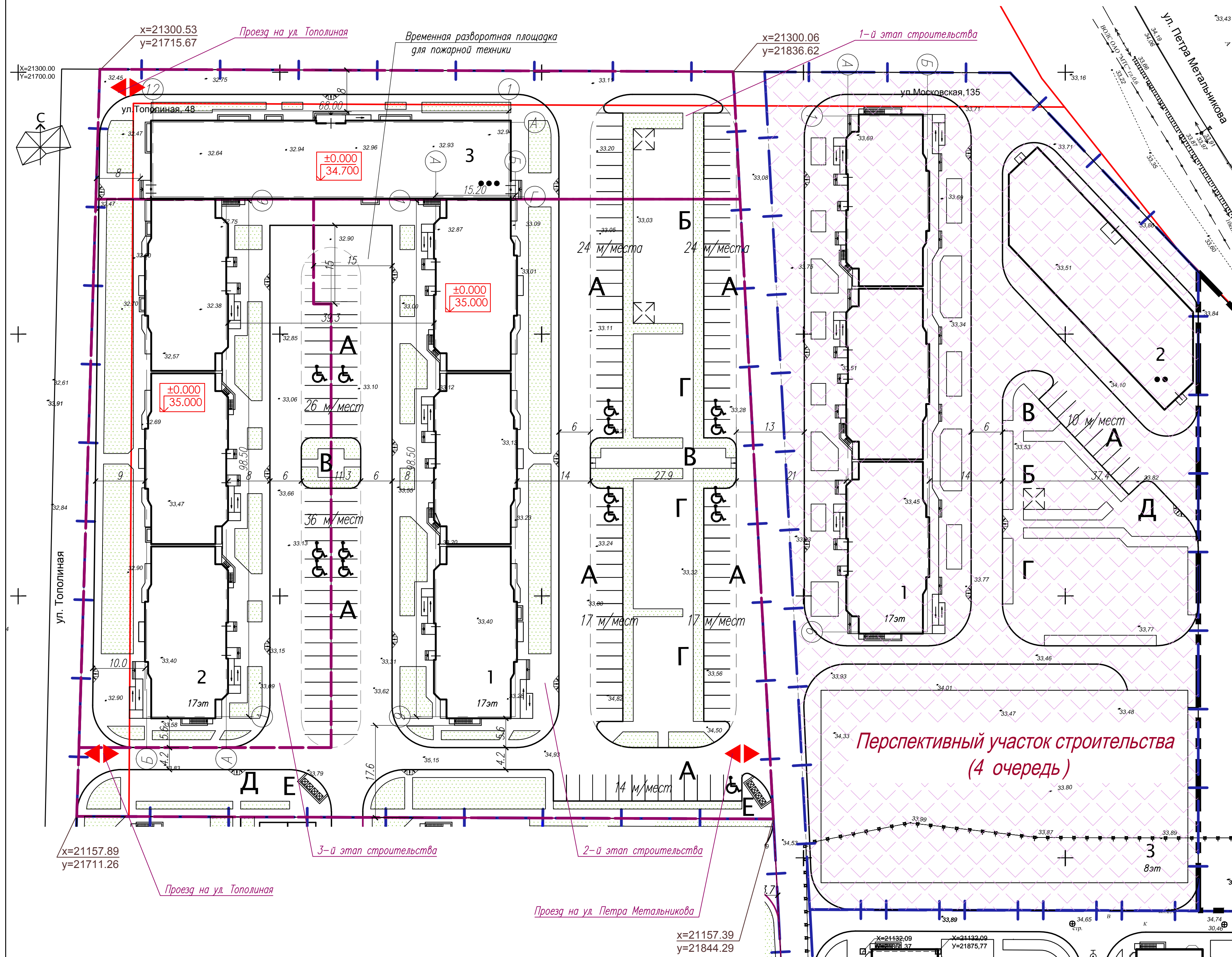
Схема планировочной организации земельного участка. М 1:500.
